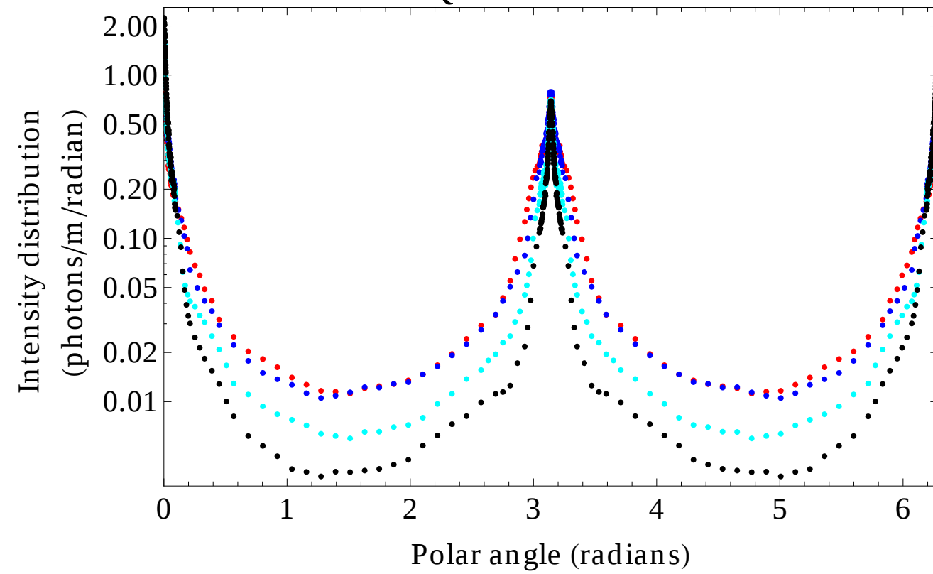
QUADRUPOLE
