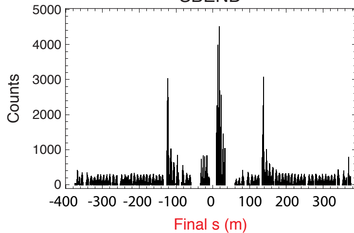
SBEND
