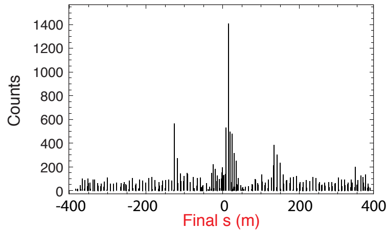
SBEND
