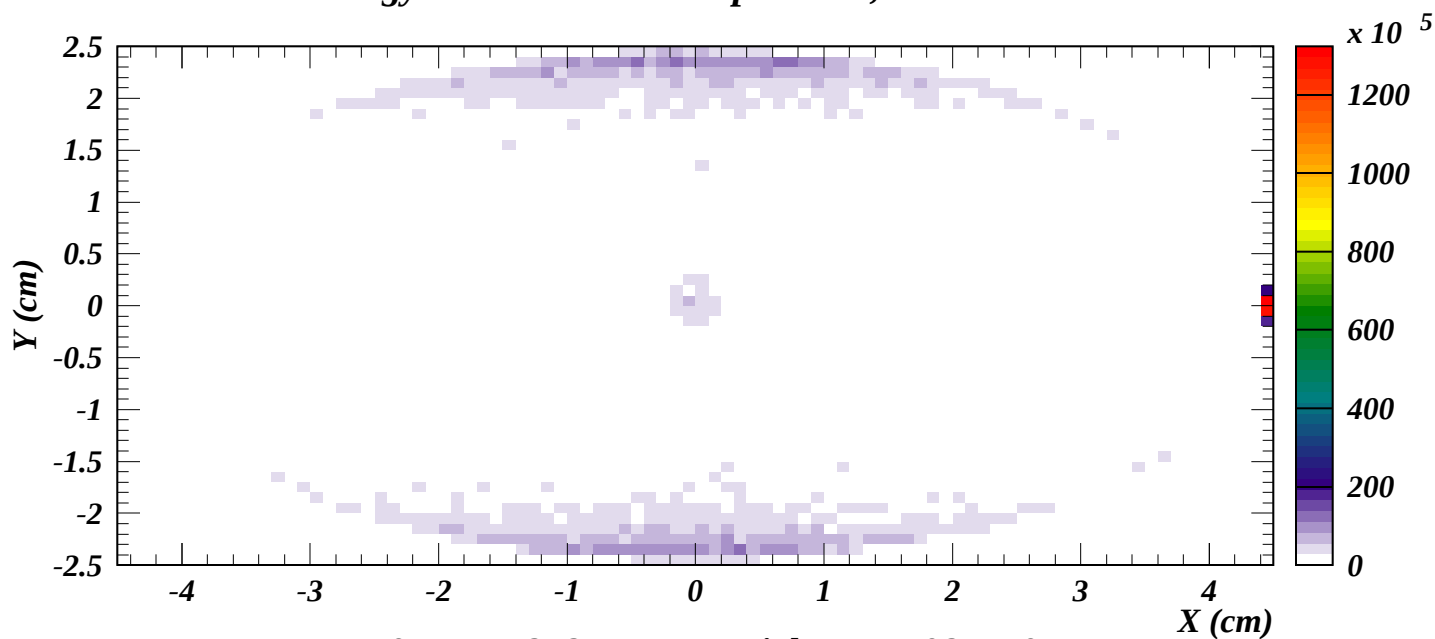
E_{kin} > 10 \text{ eV} : 64828 macroparticles, 5.54082e+09 \text{ e-}
