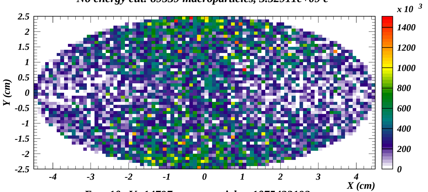
E_{kin} > 10 \text{ eV} : 14797 macroparticles, 1075432192 \text{ e-}
