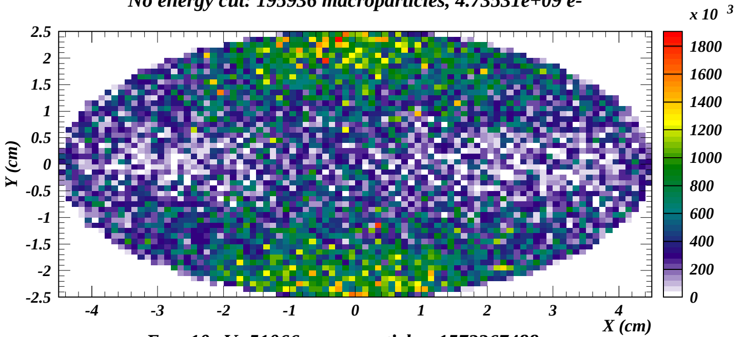
E_{kin} > 10 eV: 51066 macroparticles, 1572367488 e-
