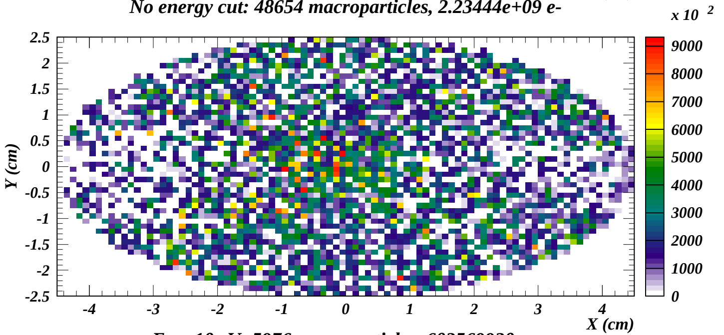
E_{kin} > 10 eV: 5976 macroparticles, 603569920 e-
