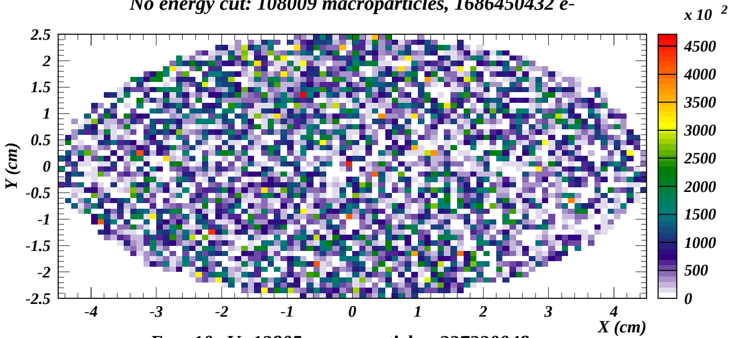
E_{\text{kin}} > 10 \text{ eV} : 12805 macroparticles, 237330048 e-
