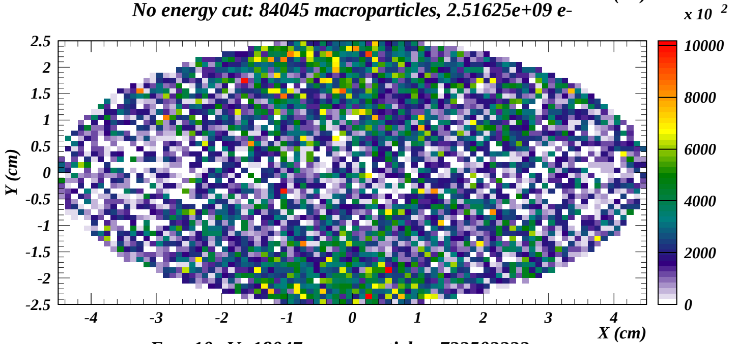
E_{kin} > 10 \text{ eV} : 18047 macroparticles, 733503232 \text{ e-}
