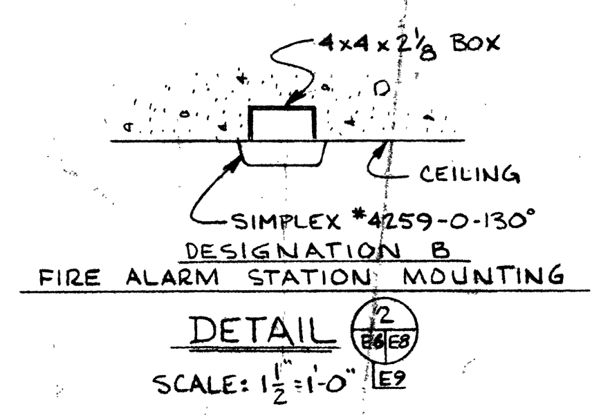
DETAIL 2 SCALE: 1 1/2" = 1'-0"
