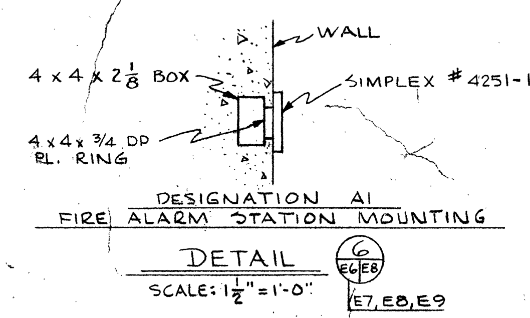
DETAIL 5 SCALE: 1 1/2" = 1'-0"
