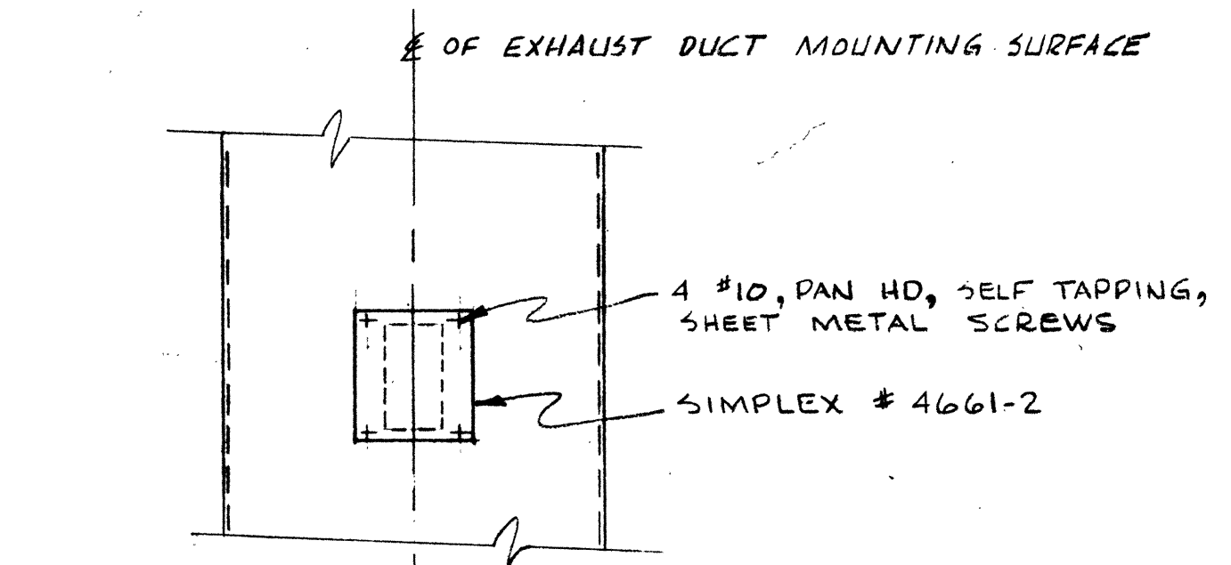
DETAIL 3 SCALE: 1 1/2" = 1'-0"
