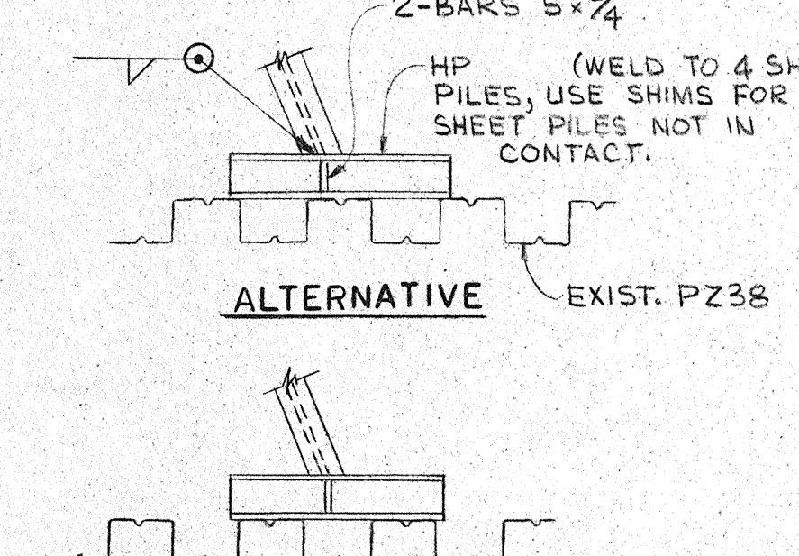
10 DETAIL SCALE: 1/2\"/>
