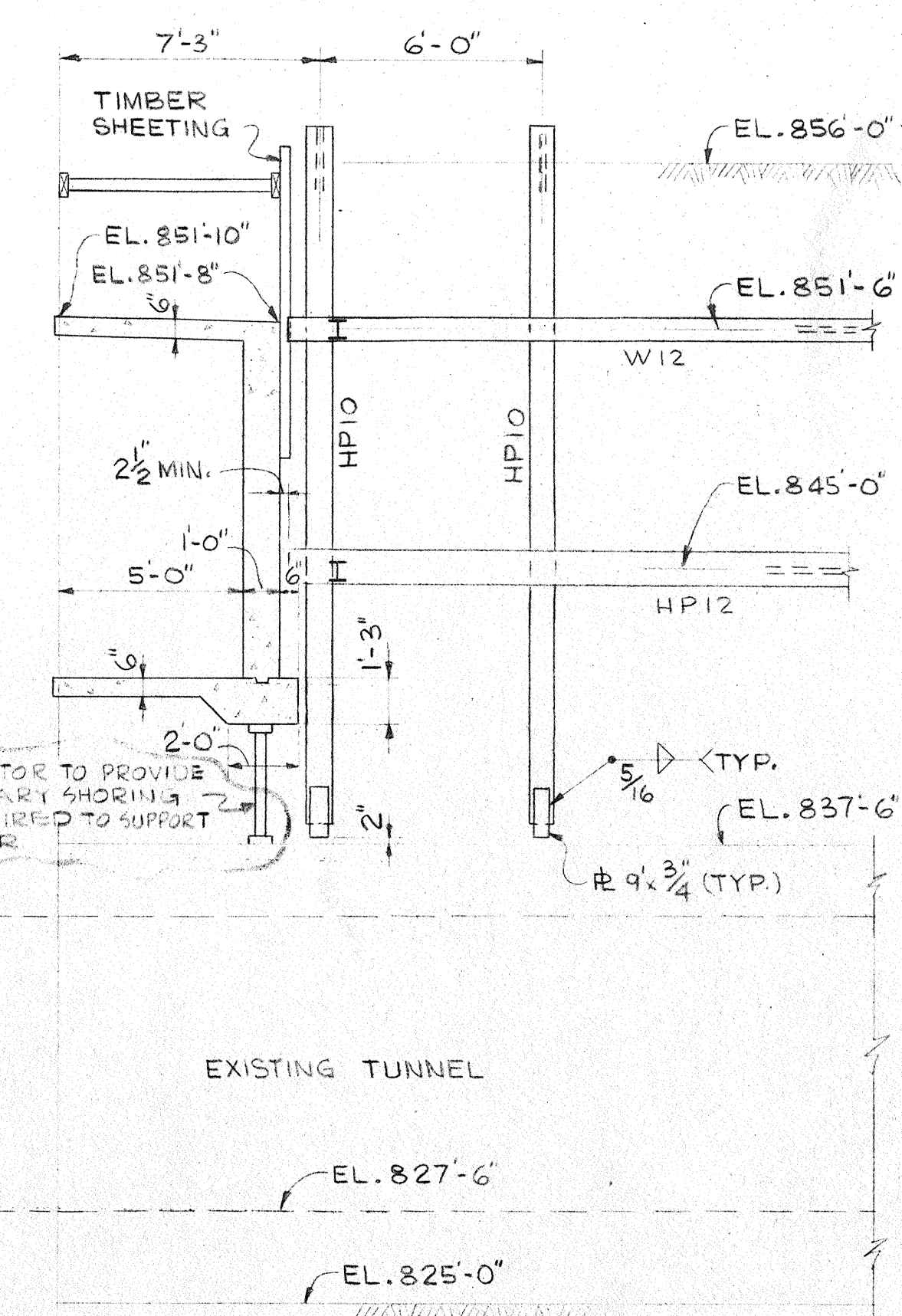
7 SECTION SCALE: 1/4\"/>
