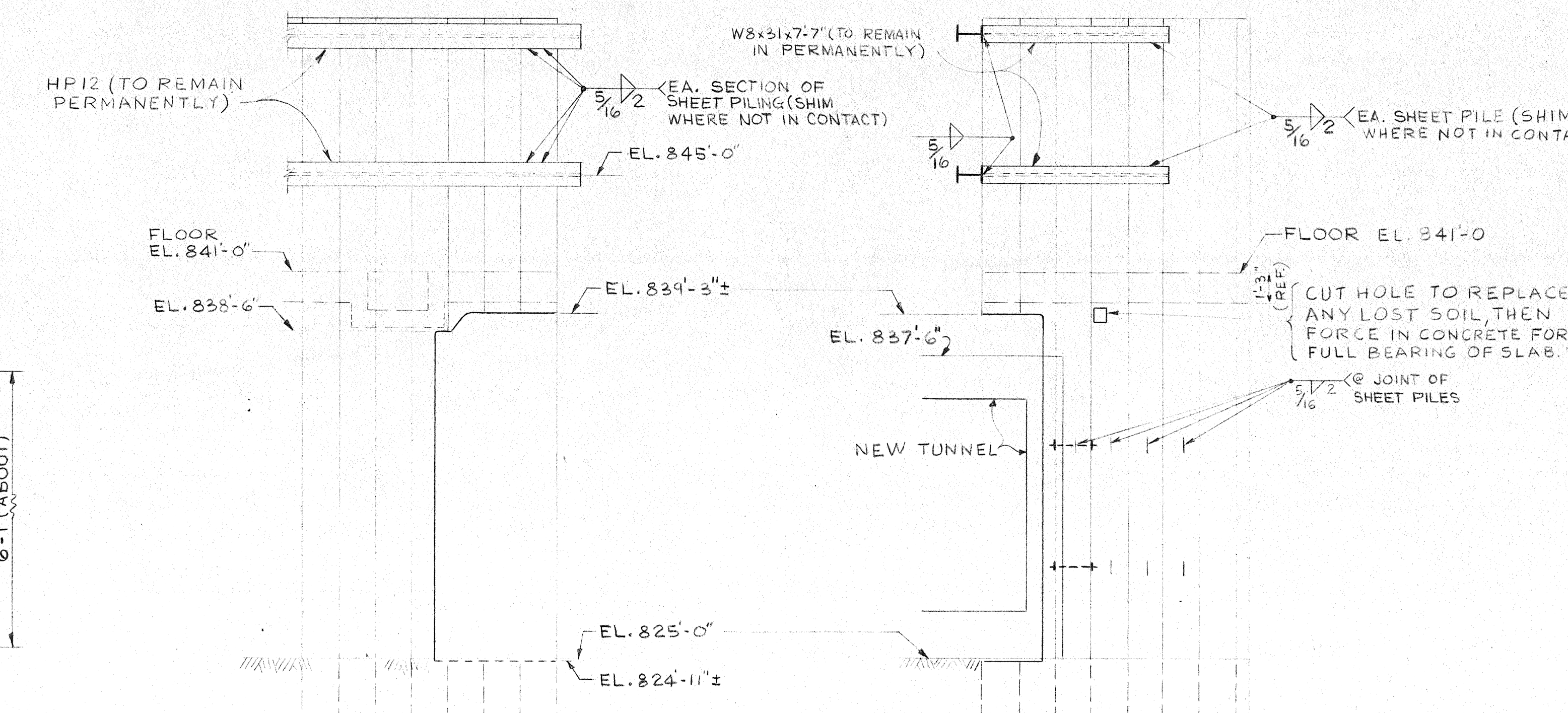
6 SECTION SCALE: 1/2\"/>
