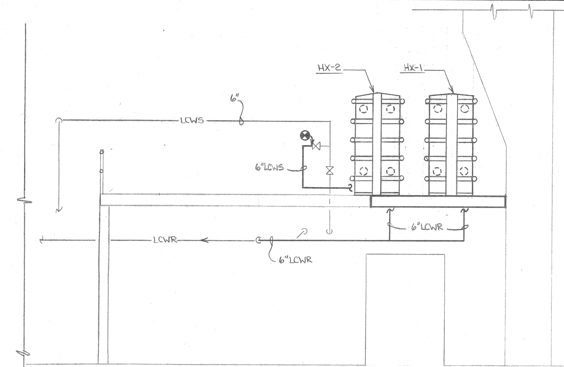
SECTION B SCALE 1/4" : 1'-0"
