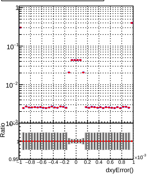
(PackedCandidate::dxyError() - reco::Track::dxyError())/reco::Track
