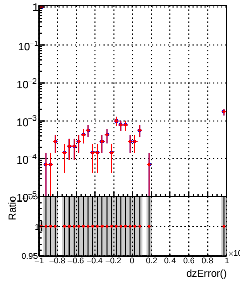
(PackedCandidate::dzError() - reco::Track::dzError())/reco::Track
