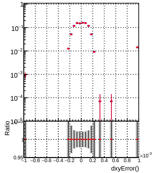
(PackedCandidate::dxyError() - reco::Track::dxyError())/reco::Track
