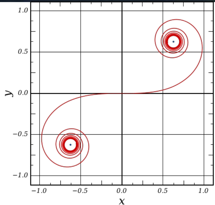
Cornu Spiral
