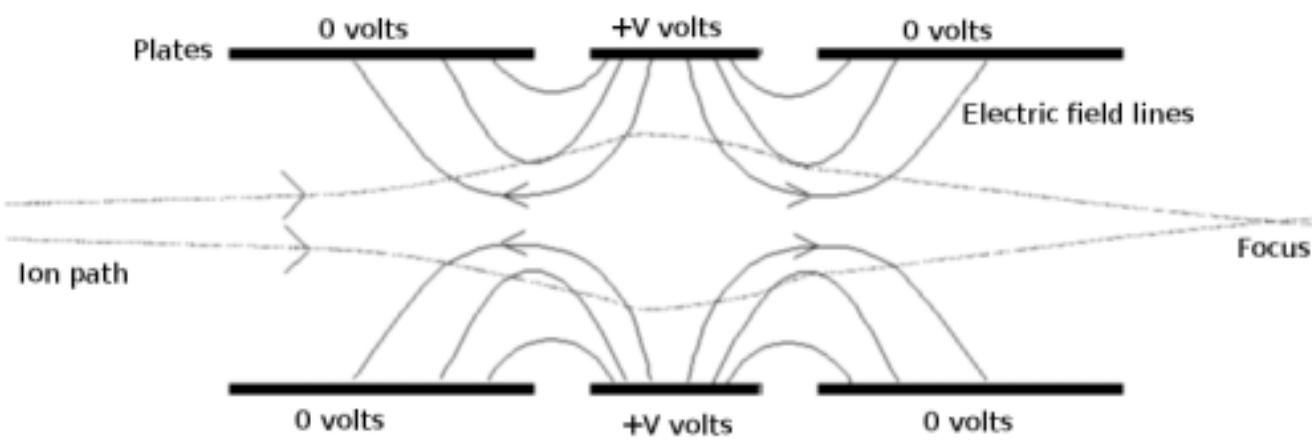
Einzel Lens
