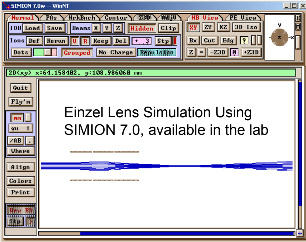
Einzel Lens
